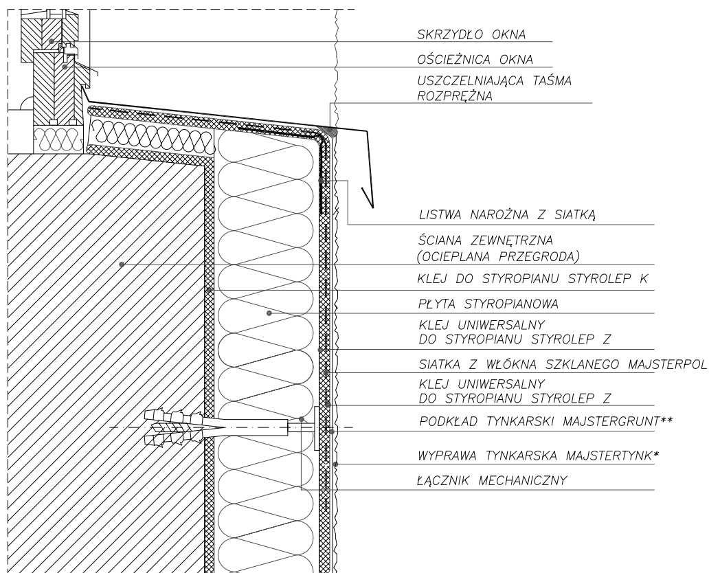
DETAL OBRÓBKI PARAPETU PRZEKRÓJ PIONOWY
